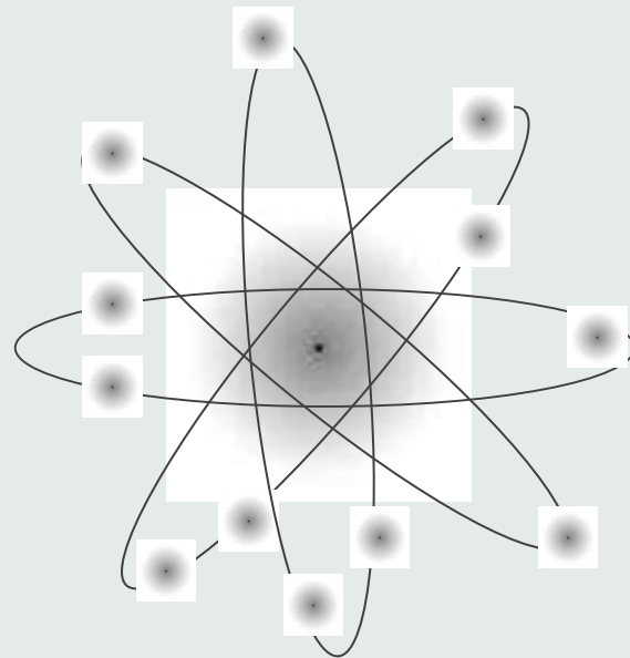
Urânio (92 elétrons)
