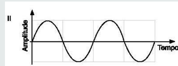
Radiação
